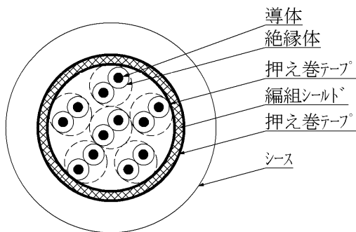
・ 6 P 断面図
