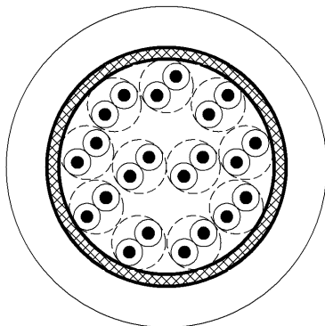
・ 11 P 断面図
