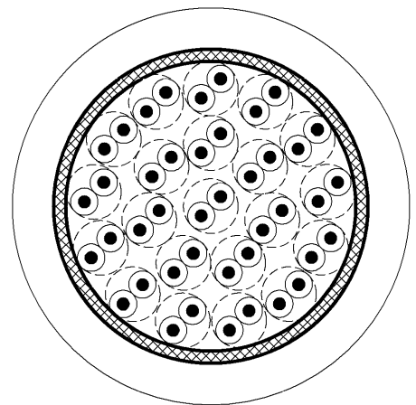
・ 21 P 断面図
