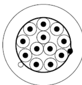
・ 12 C 断面図
