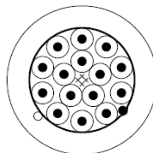
・ 15 C 断面図
