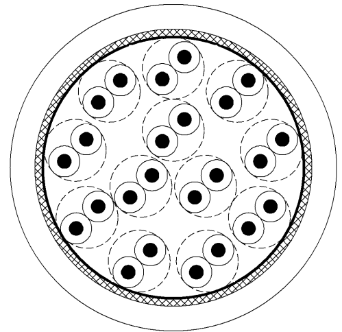
・ 12P 断面図
