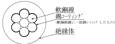
TZ形導体断面図
